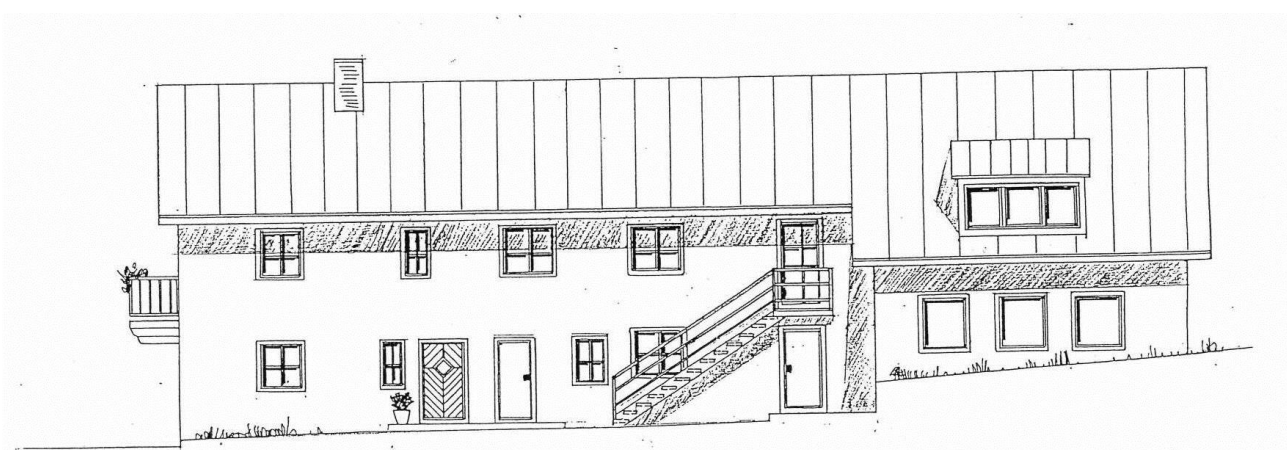
ANSICHT OSTEN:
