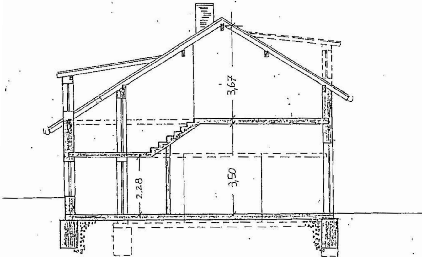
SCHNITT A-A
