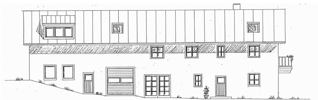
ANSICHT WESTEN
