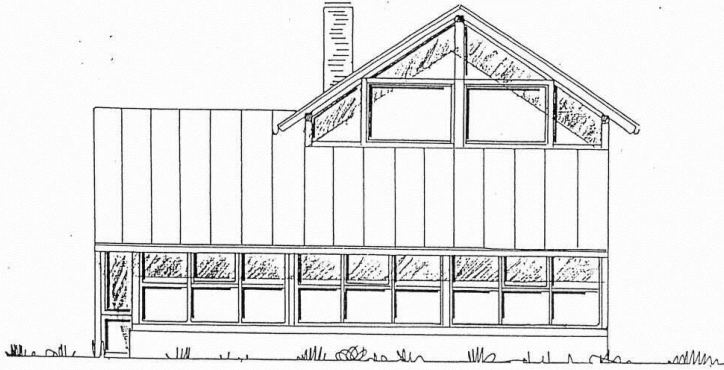
ANSICHT NORDEN
