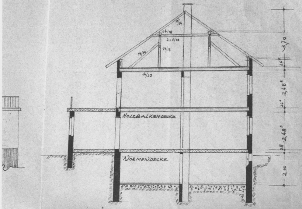
QUERSCHNITT = A B
