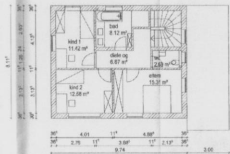
OBERGESCHOSS
