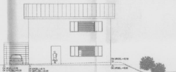
ANSICHT NORD
