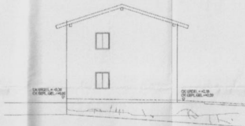
ANSICHT WEST
