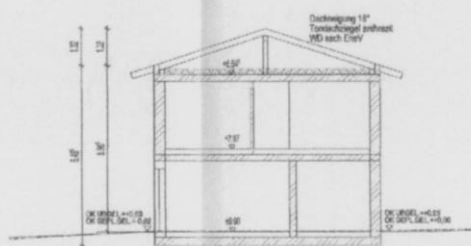
SCHNITT A-A
